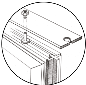
CORNICE SUPERIORE TOP FRAME
